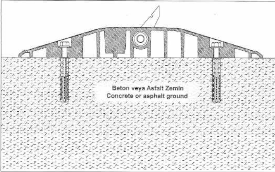
Montaj Uygulama Resmi Installation Picture
